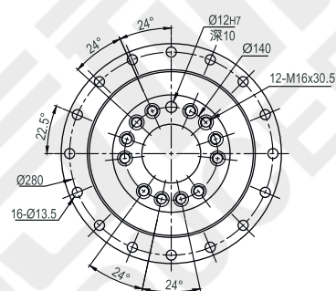
输出端/ OUTPUT
