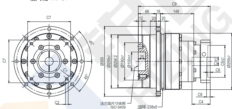
输入端/ INPUT
