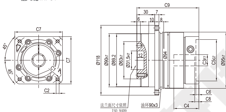
输入端/INPUT
