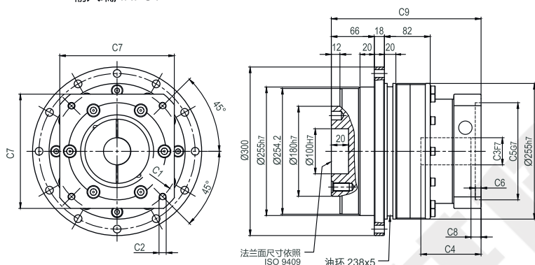
输入端/INPUT
