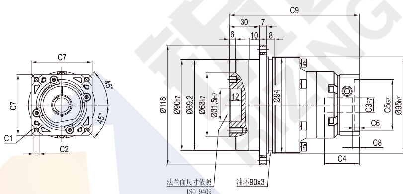
输入端/ INPUT
