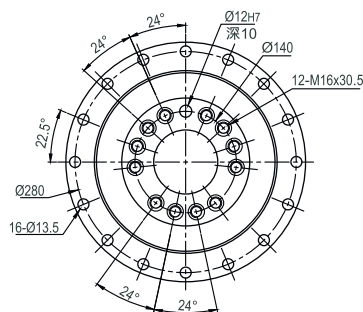
输出端 /OUTPUT
