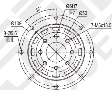
输出端/ OUTPUT
