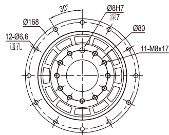
输出端 /OUTPUT
