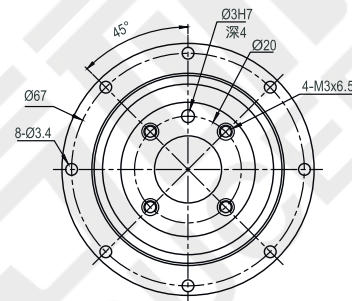
输出端/ OUTPUT
