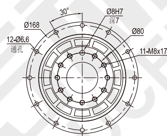
输出端/ OUTPUT
